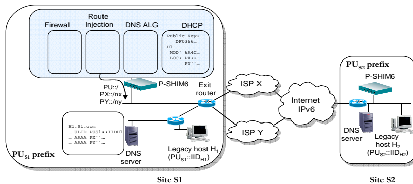
Fig. 2. Ejemplo de arquitectura basada en Proxy SHIM6 (P-SHIM6)
