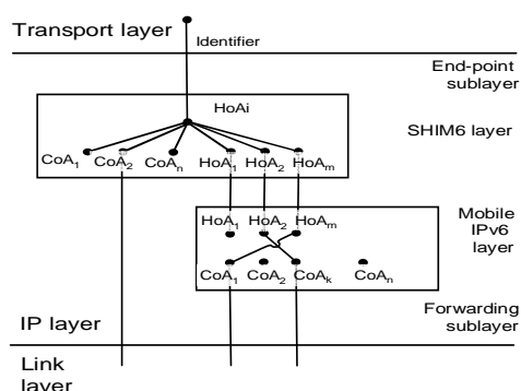
Fig. 3. Combinación de SHIM6 y MIPv6 para mejorar la tolerancia a fallos.
