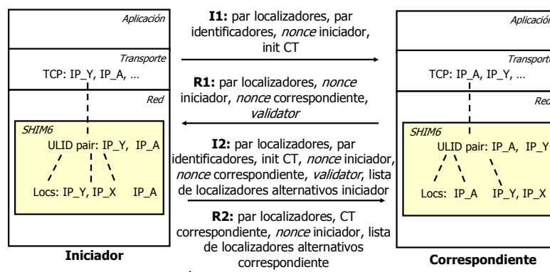
Fig. 1. Establecimiento del contexto SHIM6
